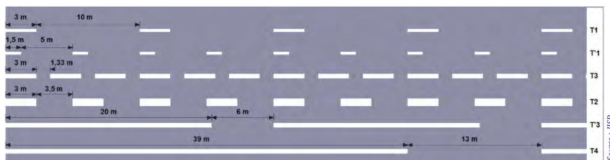
Les différents types de ligne longitudinales
