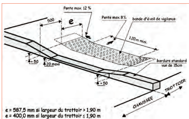
Abaissé de bordures équipé d'une BEV
