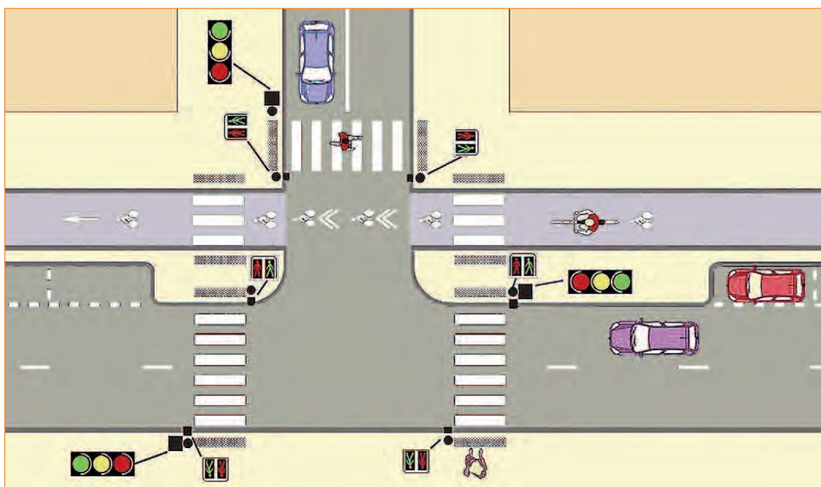
Piste cyclable traversant une chaussée dans un carrefour à feux
